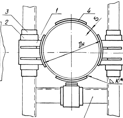
Опорная конструкция
