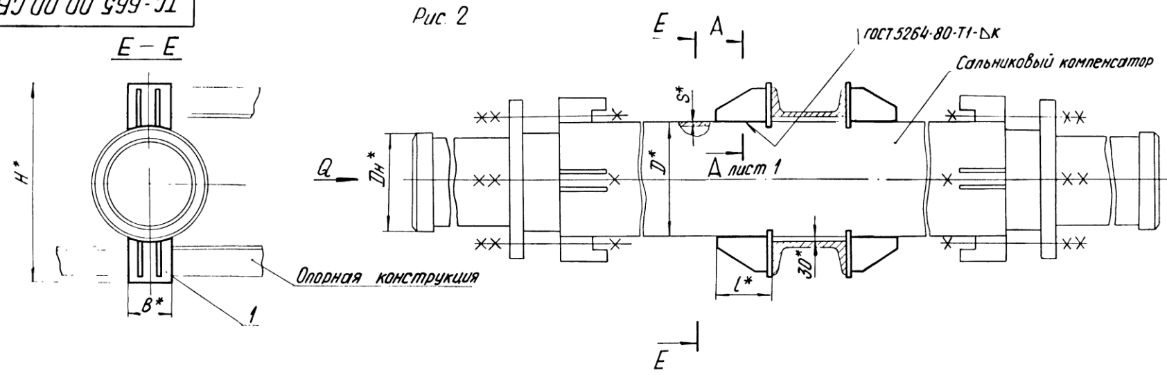
Размеры в мм
