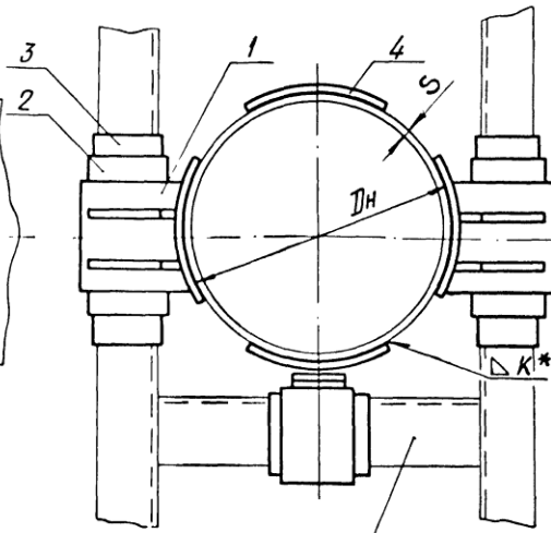
Опорная конструкция
