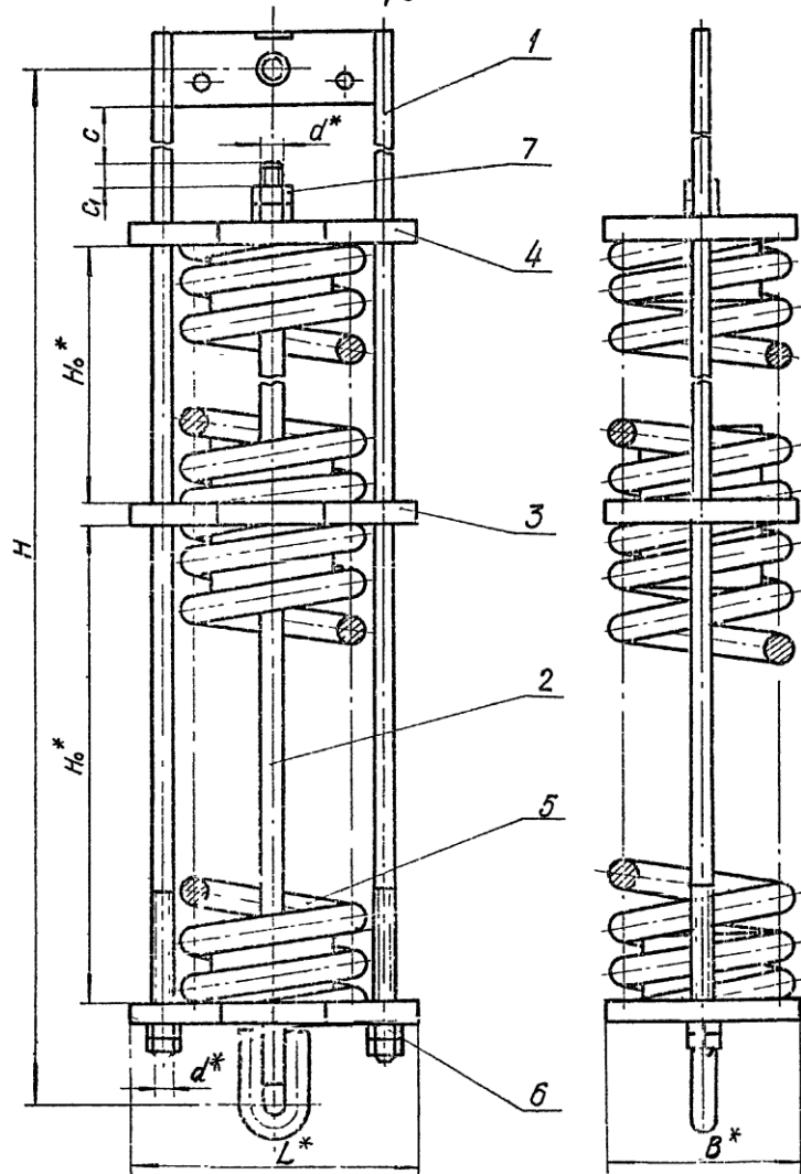
Блок пружины двойной
