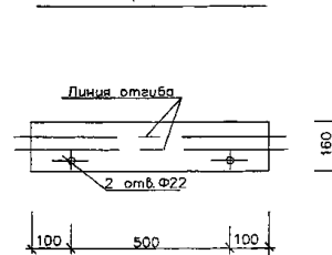
Развертка поз.10
