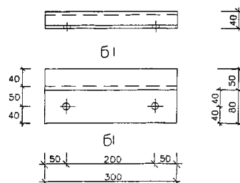
полозья поз.10
