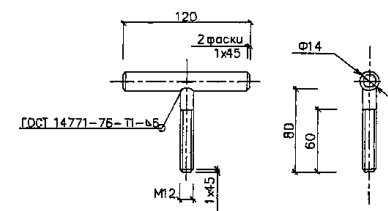
петля поз.б
