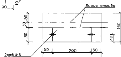
Развертка поз.10
