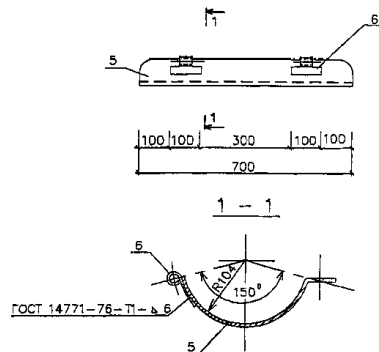
Развертка поз.5
