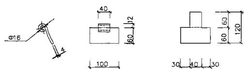
петля поз.6
