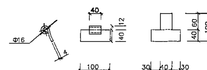
Развертка поз.10
