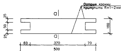
Развертка поз 9
