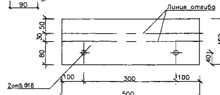
Развертка поз.10
