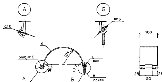
Развертка поз 9
