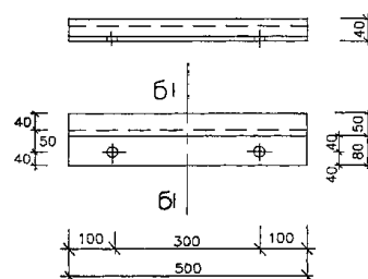
петля поз.6
