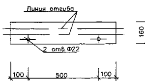
Развертка поз.10
