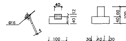
Развертка поз.10
