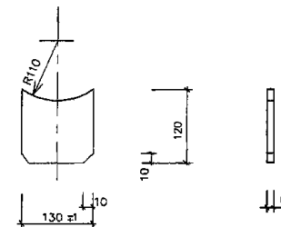
ребро поз.3
