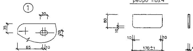
ребро поз.4
