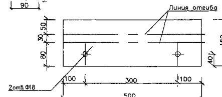
Развертка поз.10
