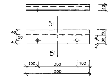
Развертка поз.6
