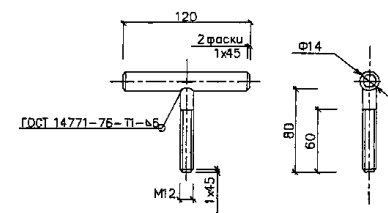
петля поз.6
