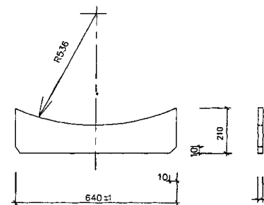
ребро поз.3
