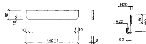
ребро поз.4
