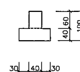
Развертка поз.6
