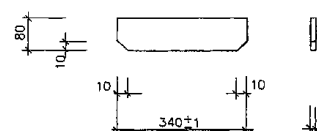
ребро поз.4
