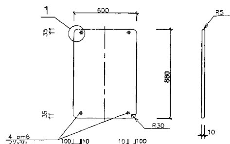
опорная плита поз.1
