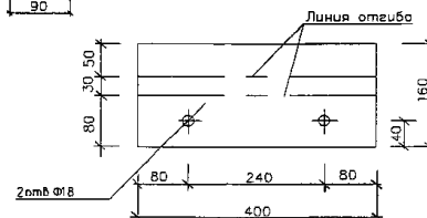
Развертка поз.10
