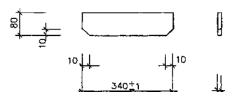
ребро поз.4
