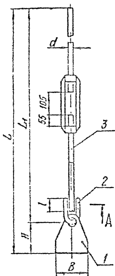
Исполнение 1
