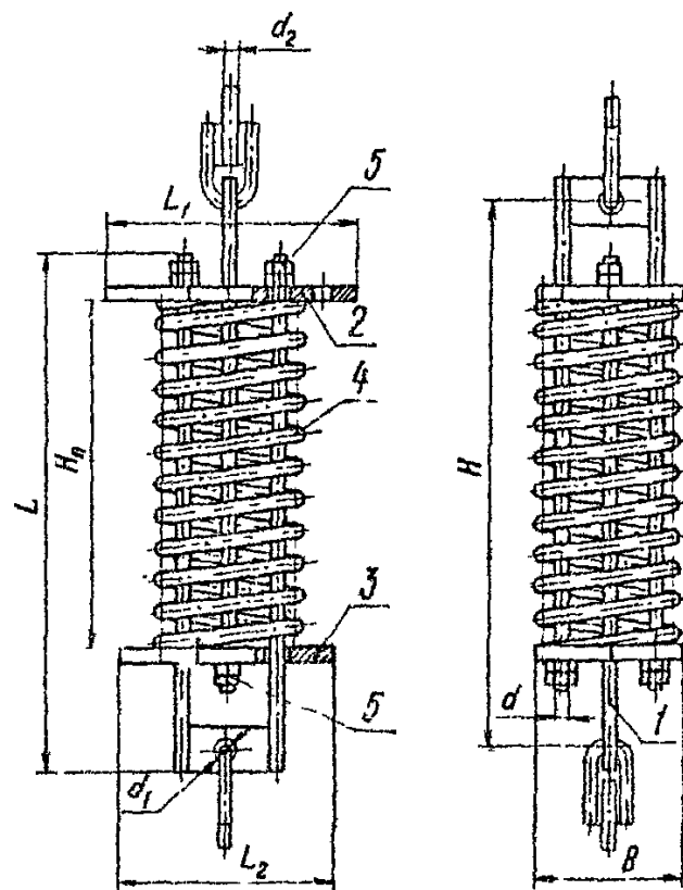
1 — траверса с тягами, 2 — основание верхнее, 3 — основание нижнее; 4 — пружина; 5 — гайка
