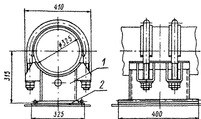
1 — опора скользящая 325 ОСТ 108.275.32—80; 2 — плита направляющая 325 ИОСТ 108.275.41—80
