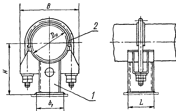
1 — опора однохомотовая; 2 — прокладка
