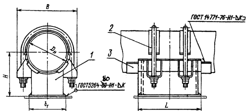
1 — опора двухкомуровая; 2 — прокладка; 3 — упор
