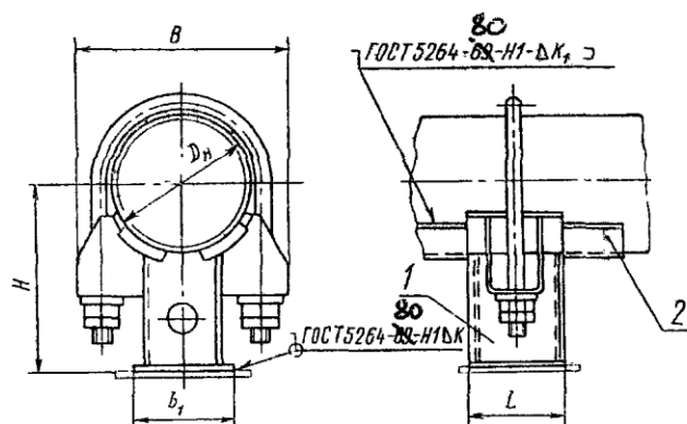
1 — опора одноконцовая; 2 — упор
