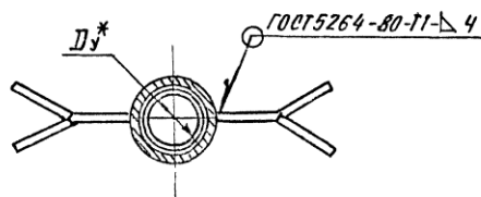
А - А
