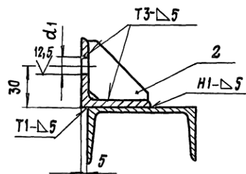
A-A (1:2)
