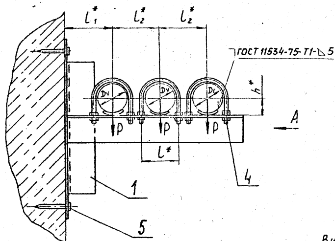
Вид А
