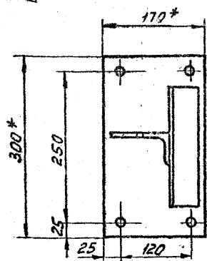
Вид А
