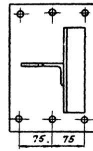
Рис 2 Вид А Остальное см. Рис. 1
