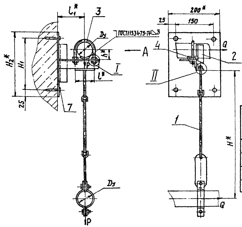
Вид А
