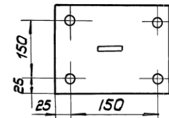
Рис. 4 Остальное - см. рис. 1 М 1:5
