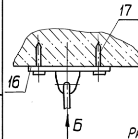
Рис. 3 Остальное - см. рис. 1 М 1:5
