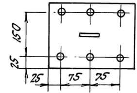
Рис.4 ОСТАЛЬНОЕ - СМ. РИС.1 М1:5
