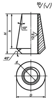
Рисунок 15 — Коническая втулка (поз. 16 на рисунке 1)
