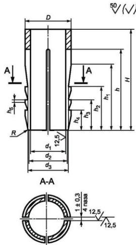
Рисунок 14 — Разжимная цанга (поз. 15 на рисунке 1)
