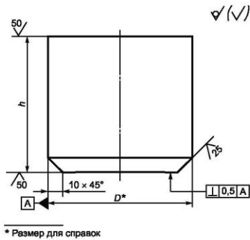
Рисунок 12 — Втулка (поз. 2 на рисунке 10)
