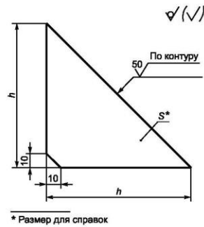
Рисунок 11 — Ребро (поз. 1 на рисунке 10)
